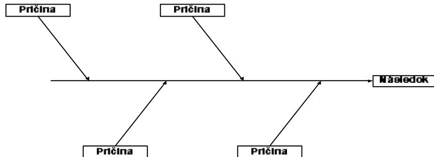
Obrázok 1 Ishikawov diagram
