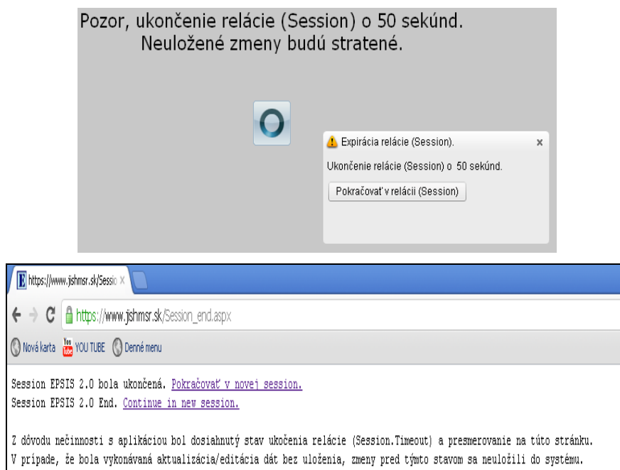
Obrázok 5 Ukončenie relácie
